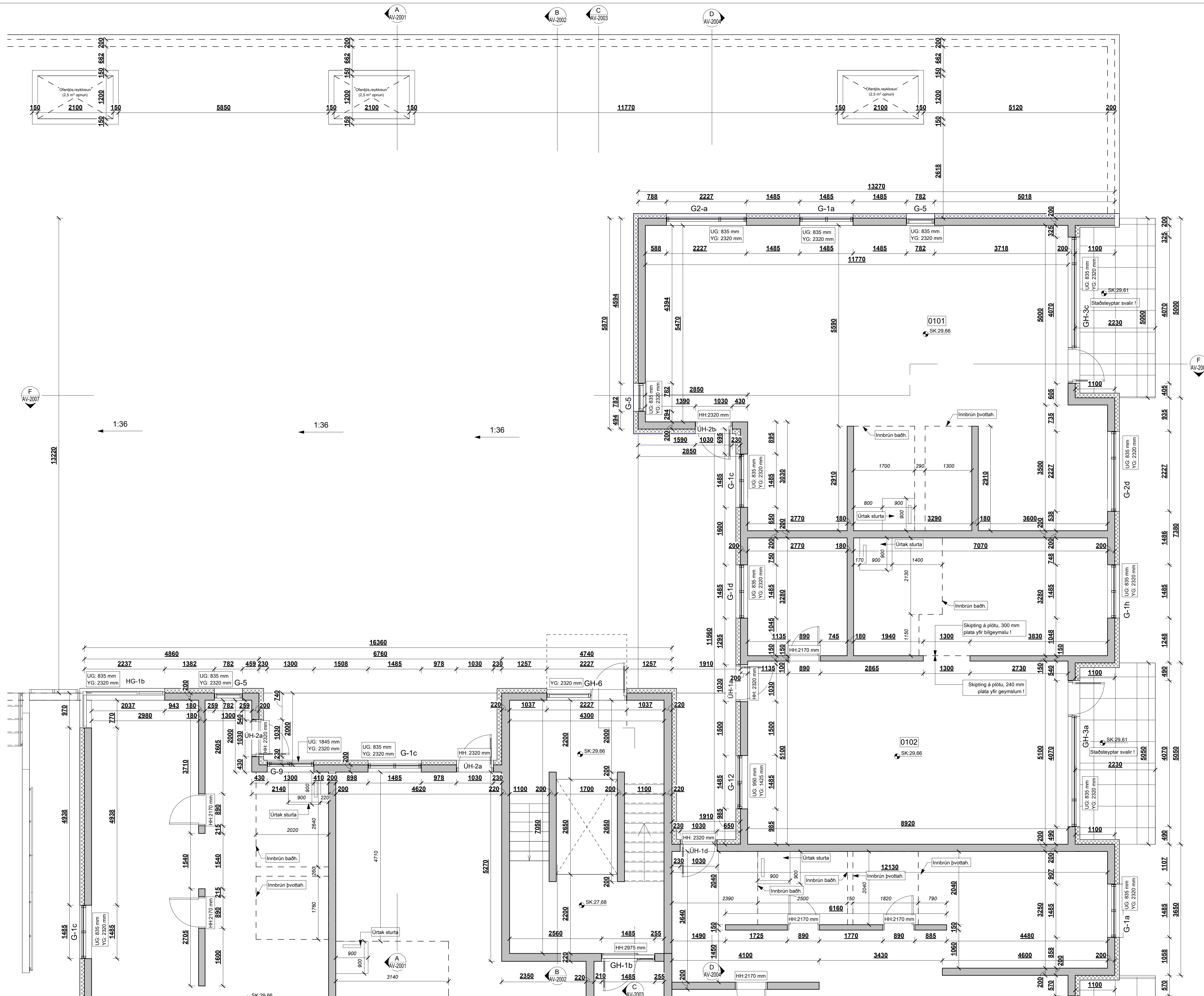
1.HÆÐ - STEYPU TEIKNING - B mkv: 1 : 50
