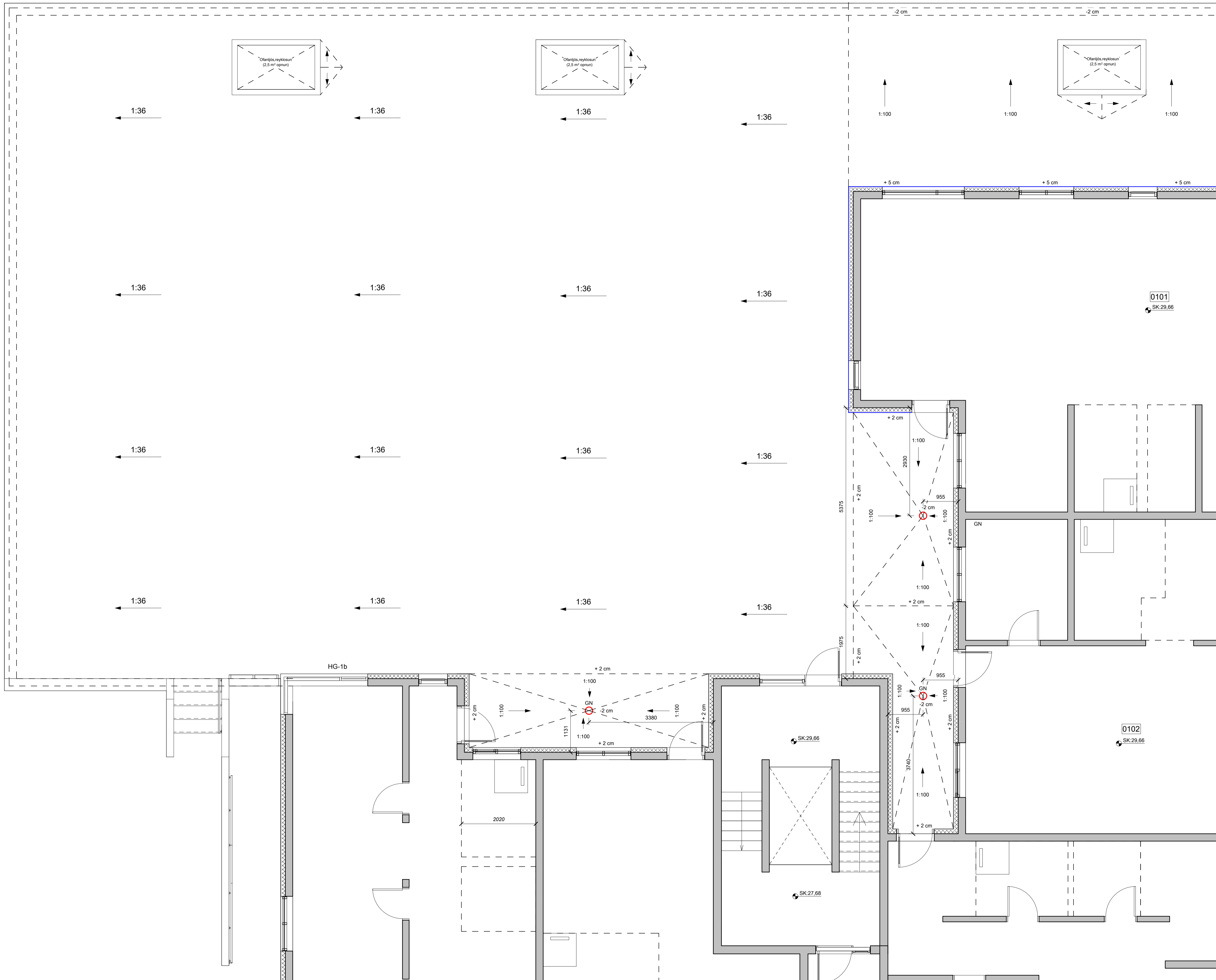
1.HÆÐ - VATNSHALLAPLAN - A mkv: 1 : 50
