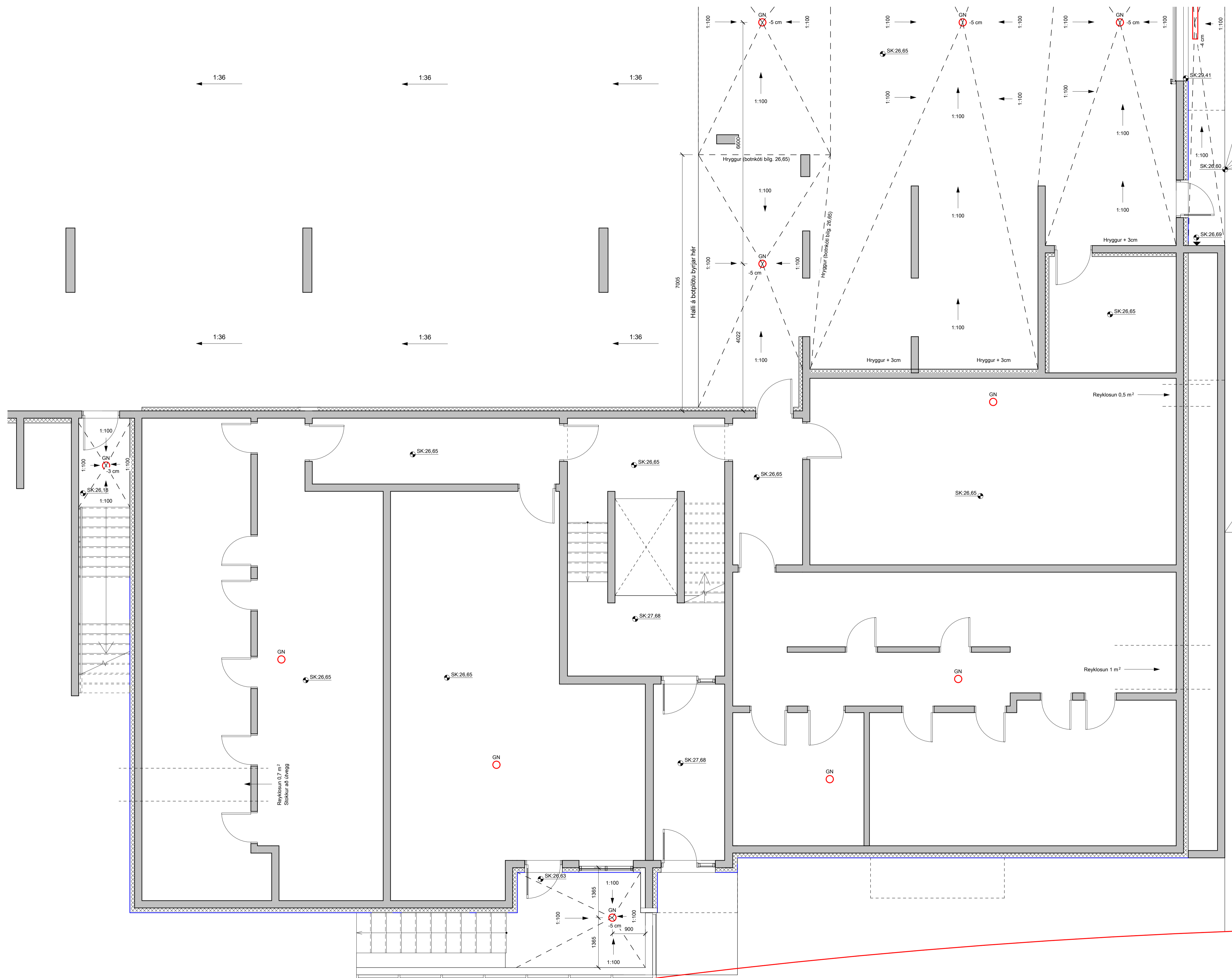
O.KJALLARI - VATNSHALLAPLAN - C mkv: 1 : 50
