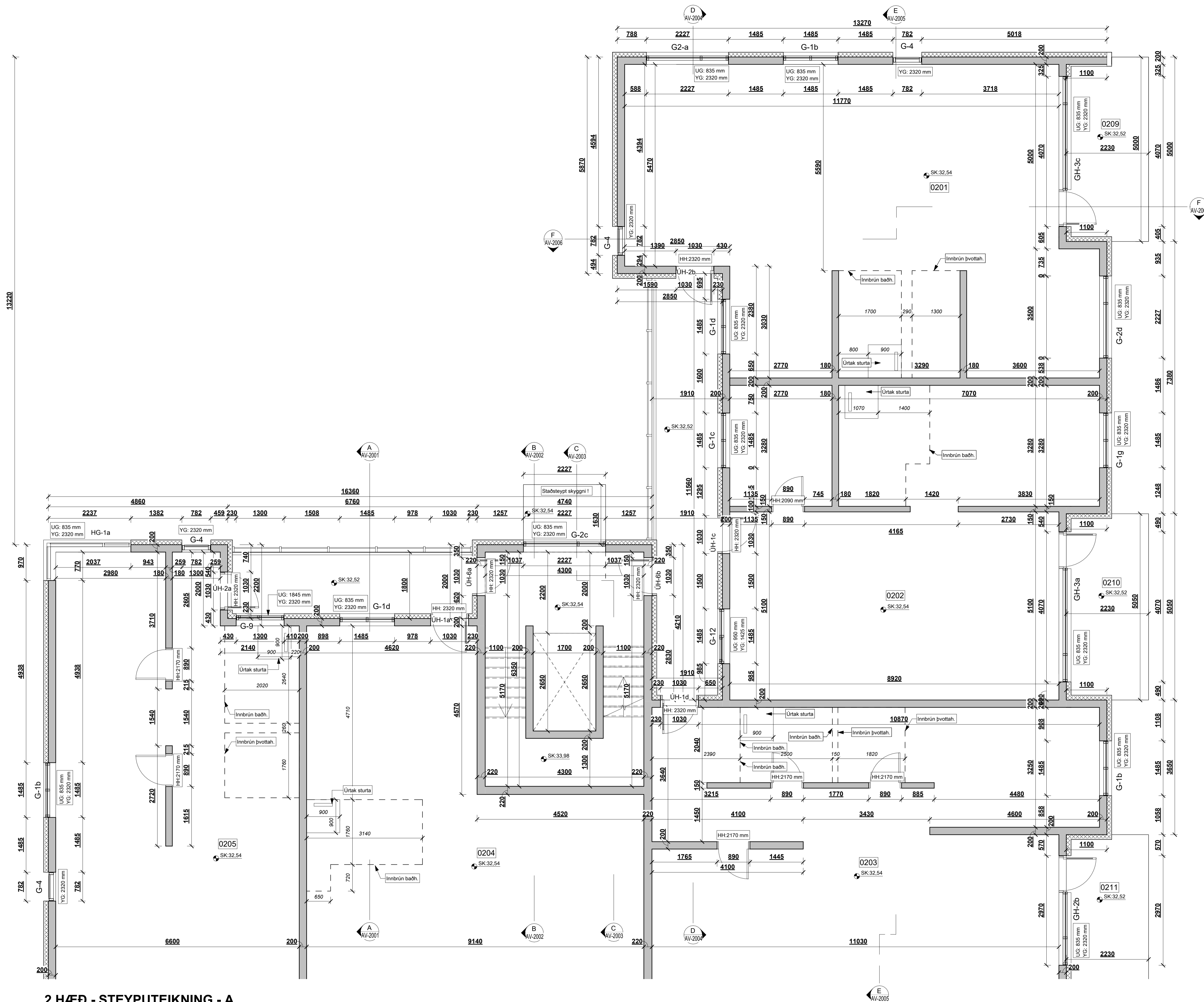
2.HÆÐ - STEYPU TEIKNING - A mkv: 1 : 50
