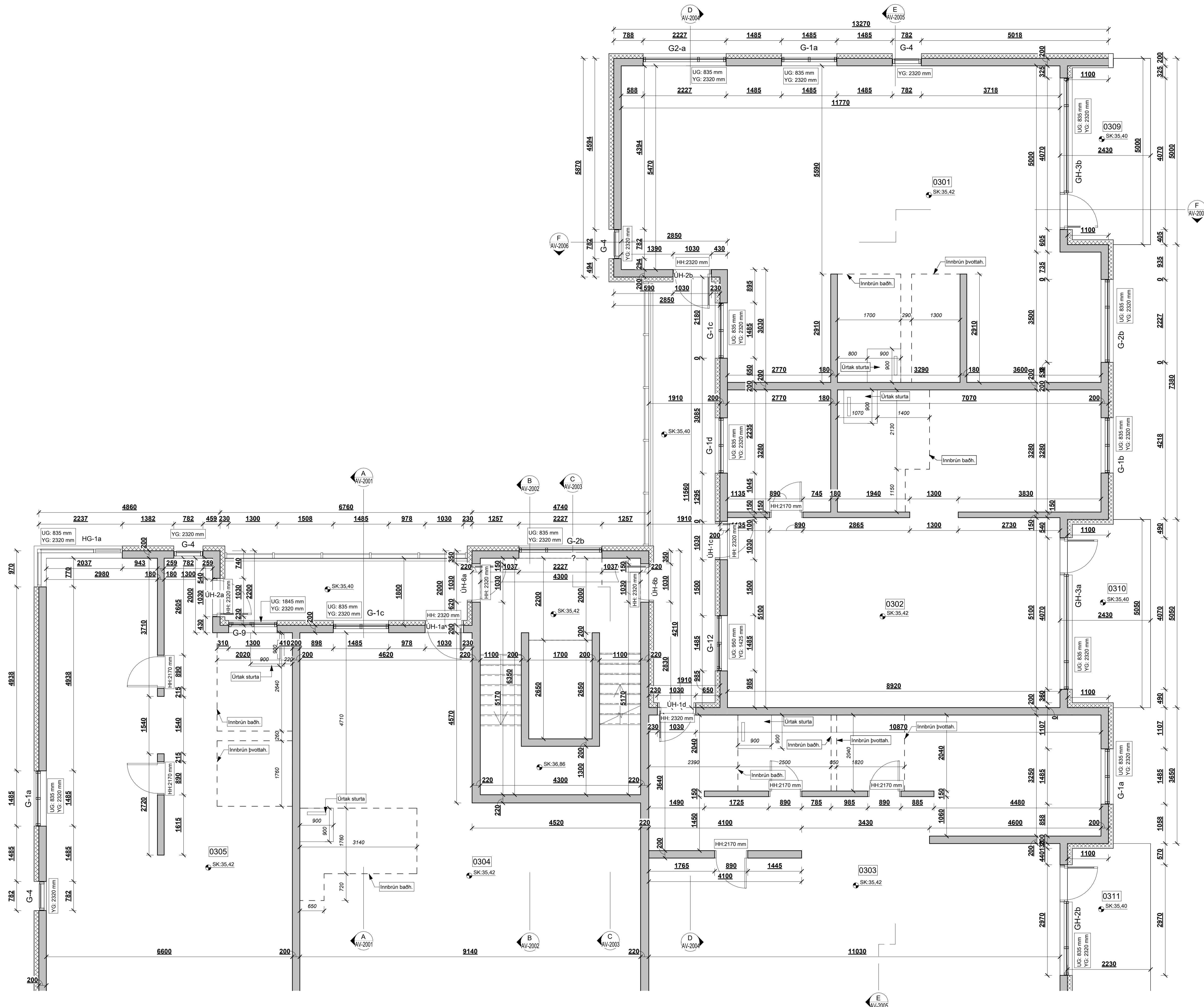
3.HÆÐ - STEYPU TEIKNING - A mkv: 1 : 50
