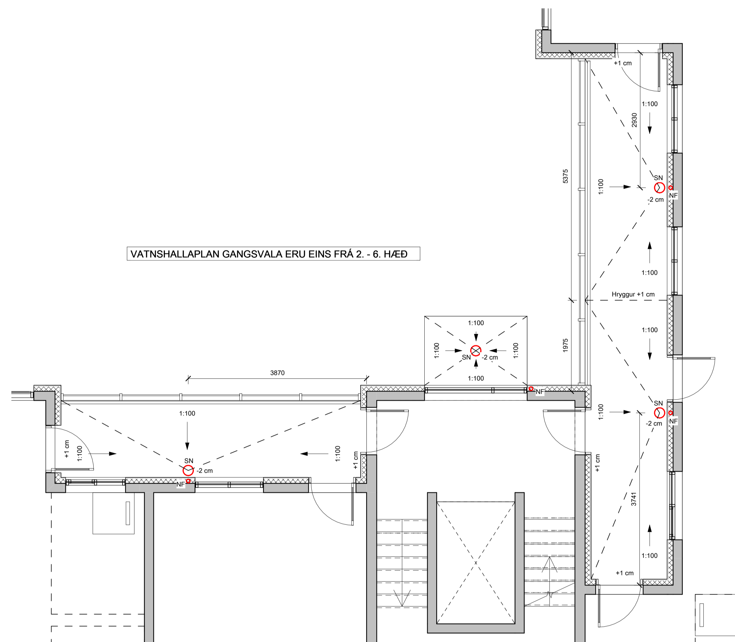
2. - 6. HÆÐ - VATNSHALLAPLAN mkv: 1 : 50
