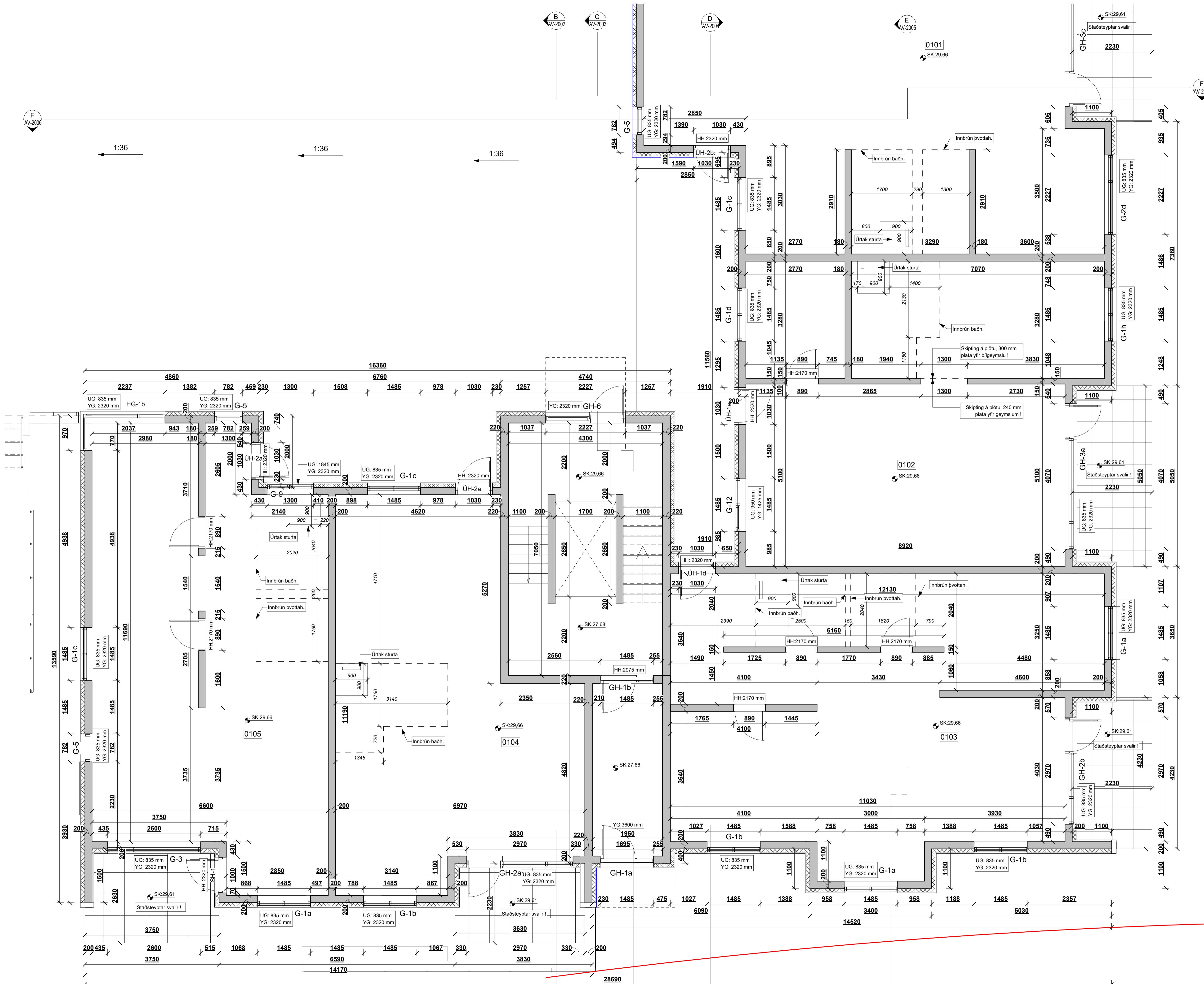
1.HÆÐ - STEYPU TEIKNING - C mkv: 1 : 50
